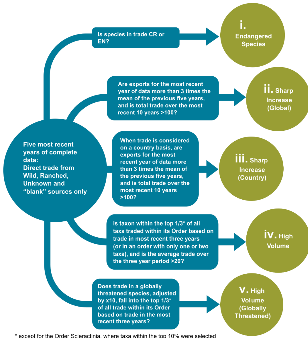
Figure 1. Schéma pour la procédure de sélection des espèces candidates à étudier dans le cadre de l'Étude du commerce important.
