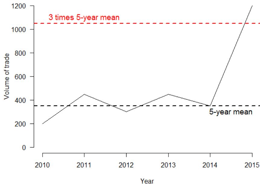
Figure 2. Illustration de l'application du critère de "forte augmentation" (exportations brutes directes).
